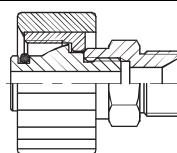
7071 Sirgühendus kõrgsurvepesurile M sk – G vk
