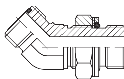
7732 Suunatav nurkliitmik 45° ORFS vk – G vk 0-rõngaga
