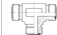
7703 T-kolmikühendus ORFS vk – ORFS vk – ORFS vk
