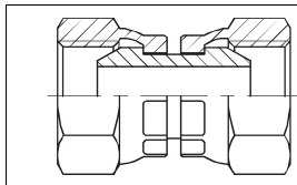
7007 Mutritega sirgühendus G sk – G sk
