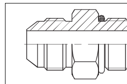
7613 J GE Sirgühendus – G vk O-rõngaga
