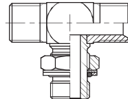
7413 Suunatav T-kolmikühendus G vk – G vk – G vk
