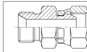
7007 Mutritega sirgühendus G sk – G sk
