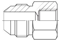
7680 J MAV Sirgühendus manomeetrile
