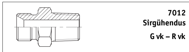
7010 Ahendav liitmik G vk – G sk lühike
