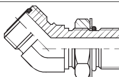
7733 Suunatav nurkliitmik 45° ORFS vk – UNF vk SAE-O ühendusega
