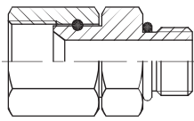
7667 J EVGE Sirgühendus JIC 37° sk – UNF vk Mutri ja O-rõngaga
